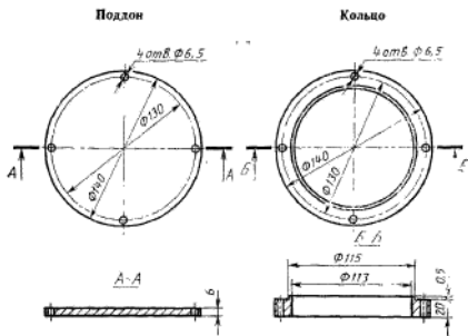
Детали формы для определения поверхностного водопоглощения
