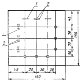
1—риски до испытания; 2—риски после испытания
