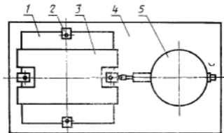
1—образец; 2—зажим; 3—прижим; 4—основание; 5—индикатор часового типа
