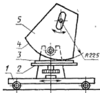
1—площадка; 2—стол; 3—образец; 4—шлифовальная шкурка; 5—рабочий элемент
